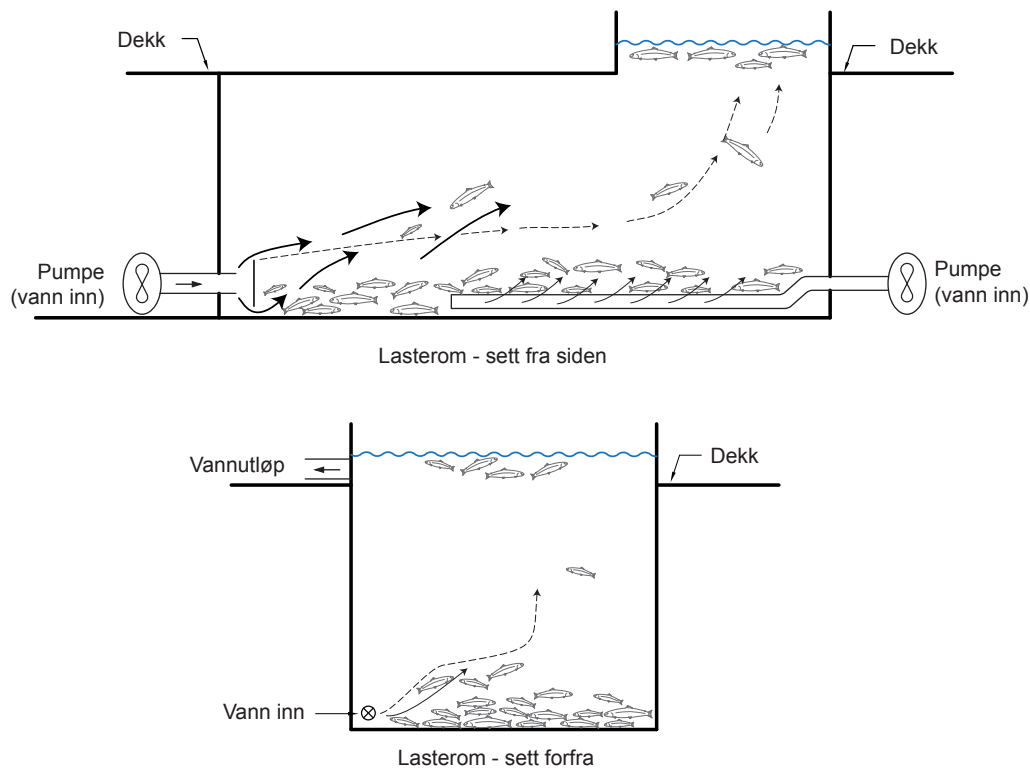
Bilde 40: Illustrasjon av vannfordeling i rom med tradisjonell vannfordeling.
